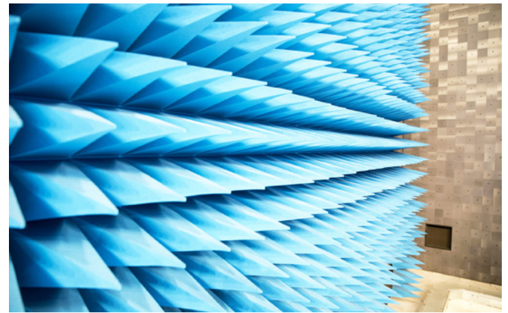
Zkouška kvality. Gigantická komora EMC pro testování elektromagnetické koexistence vozidel a jejich elektronických přístrojů a vybavení. Foto ČTK/Kryštof Kříž
